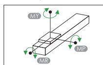
靜態容許負載慣量 Static Loading Moment
