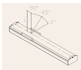
水平安裝應用 (單位:mm) Horizontal use
