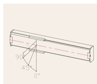
牆面安裝應用 (單位:mm) Wall installation use
