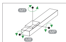
靜態容許負載慣量 Stdc Loading Moment
